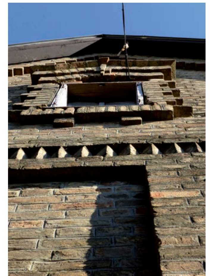
Jobbra: pajtahomlokzat-részlet; lakóházoromfal-részlet
