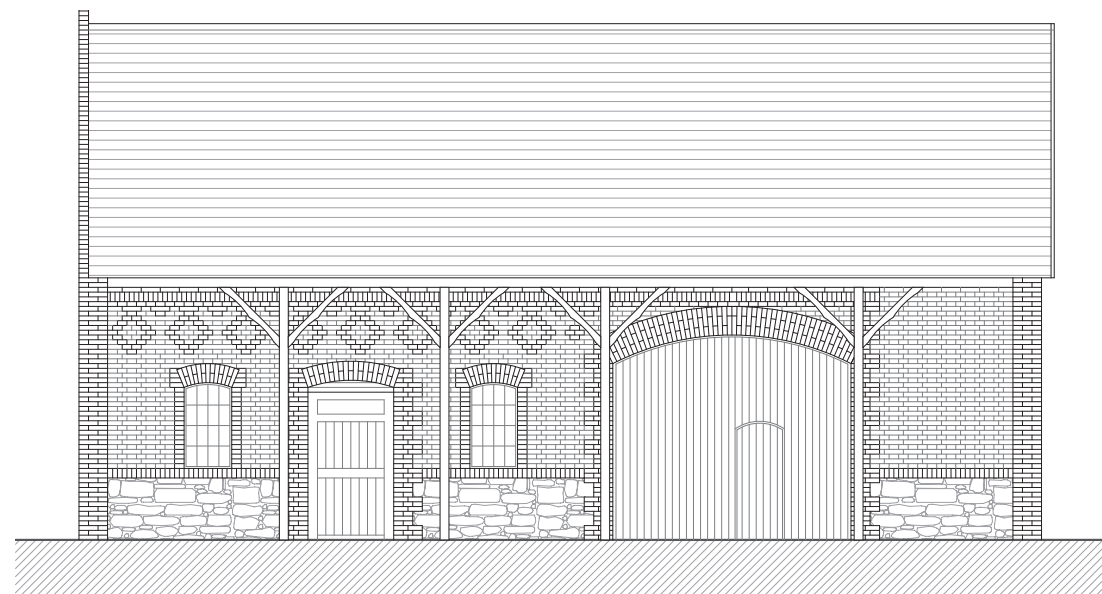
Fenn: tornácos pajta és rajzolt homlokzata
