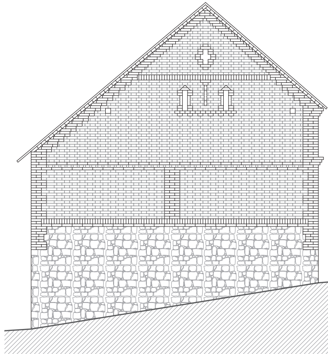
Pajtavéghomlokzat rajzolt képe
