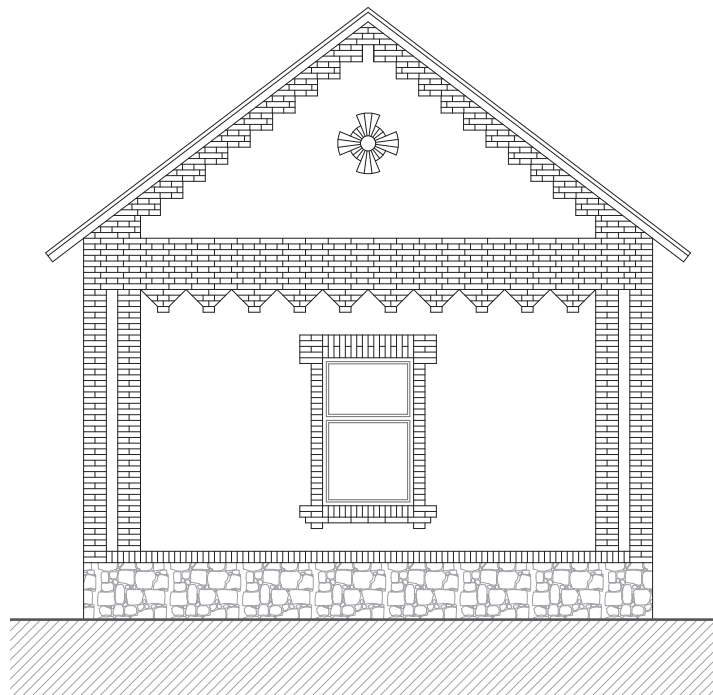
Posta rajzolt homlokzata
