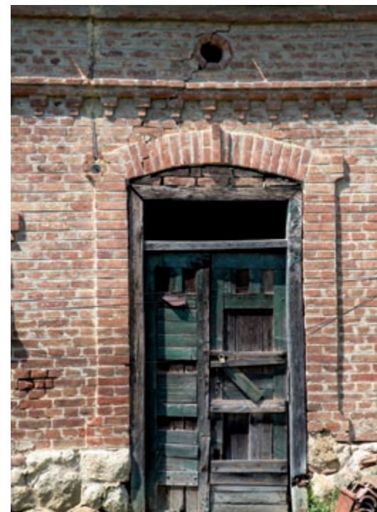
Szemben fentről lefelé: pajta; gazdasági épületek hátsó homlokzata; pajtahomlokzat-részlet; pajta Fenn: istállóajtó Jobbra: oromfal csatornával, részlet; pajtakapurészlet Lenn: Vázsnok rajzolt térképe
